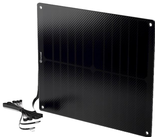
MSF15W12V 15W | 12V Dim.: 300 x 256 x 3 mm
