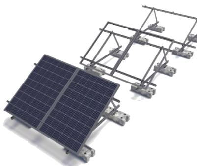
SOLSTAND TM fijación en contrapesos
