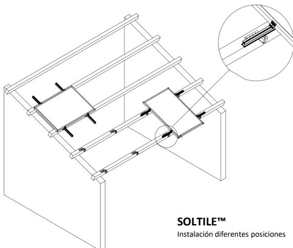
SOLTILEFIXM10 Pack 4 unidades Incluido Con junta EPDM
